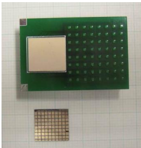
Diode Array (8x8)
